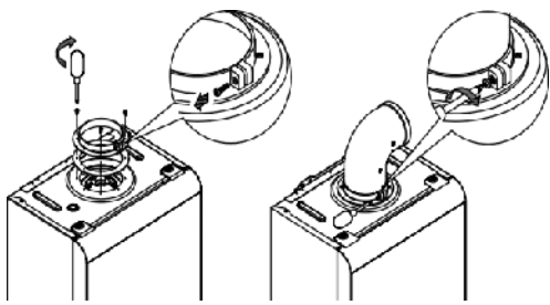
Figura 28: Instalación del conjunto de piezas
