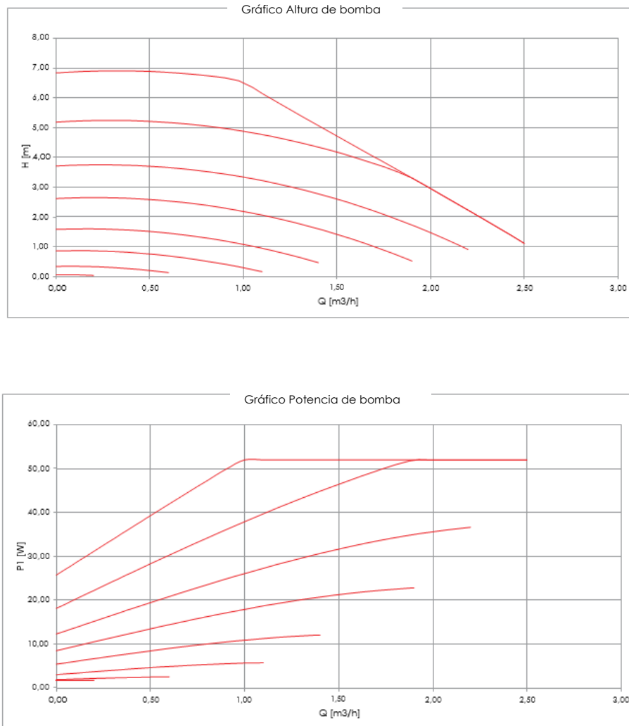
Figura 8: Gráficos de altura y potencia de bomba MINERWA
