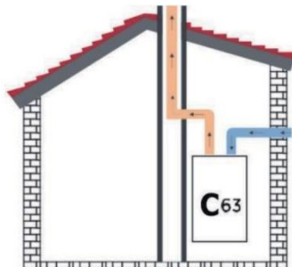
Figura 22 Descarga de humos en conducto independiente por la chimenea del edificio y aspiración de aire desde el exterior
