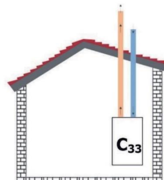
Figura 20 Instalación vertical con conductos separados. Los terminales deben estar separados 50 cm.
