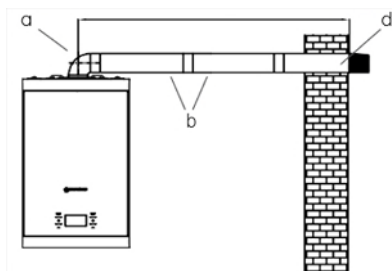
Figura 32: Instalación de chimenea simple con codo de 90°
