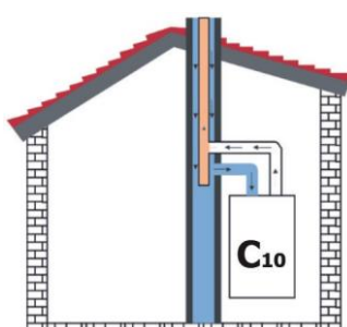
Figura 24 Descarga de humos a través de la chimenea del edificio y entrada de aire a través del conducto comunitario.
