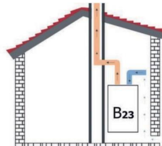
Figura 23 Descarga de humos en conducto independiente por la chimenea del edificio y aspiración de aire desde el local, mediante rejilla de ventilación.
