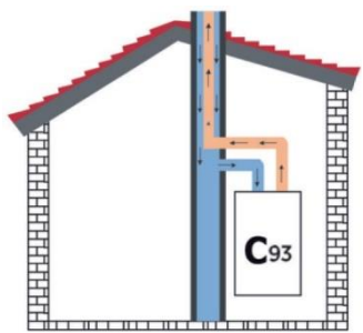
Figura 24 Descarga de humos a través de la chimenea del edificio y entrada de aire a través del conducto comunitario.
