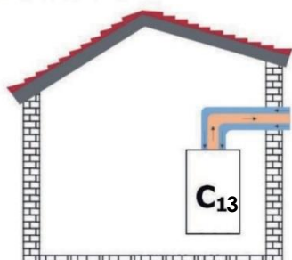
Figura 18 Descarga de humos con tubo concéntrico.
