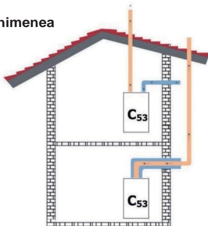
Figura 19 Descarga de humos y entrada de aire a través de tubo concéntrico. Atención: Los terminales de combustión y aspiración de aire deben instalarse en la misma orientación.
