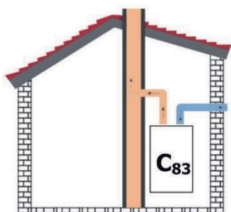
Figura 21 Descarga de humos a la chimenea del edificio y aspiración de aire desde el exterior.
